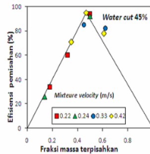
Gambar 15. Hasil efisiensi pemisahan fase tertinggi pada ( D_3/D_1=0,5 ) sudut 30^\circ L=32,99 mm W_{cut} 45%
