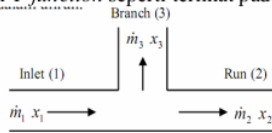
Gambar 5. Parameter aliran dua fase di T-junction (Yang dkk.,2006)
