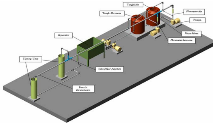
Gambar 8. Skematik instalasi penelitian
