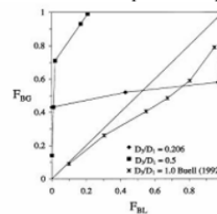
Gambar 4. Pengaruh rasio diameter terhadap Pemisahan fase pada J_L=0,0021 m/s Dan J_G=2,7 m/s (Walter L.C dkk., 1997)
