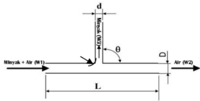
Gambar 3. Model sederhana dari T-junction
