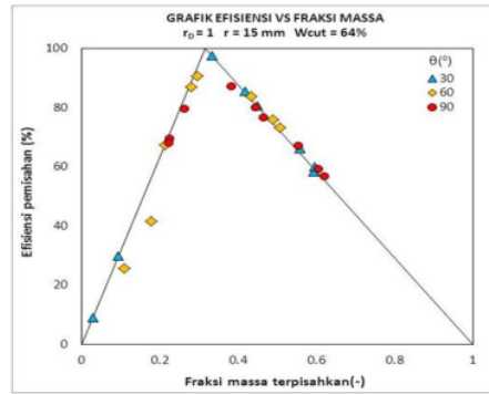
Gambar 8. Hasil Efisiensi pemisahan fase tertinggi pada ( r_D = 1 ), radius belokan 15mm, sudut 30^\circ , W_{cut} 64%.
