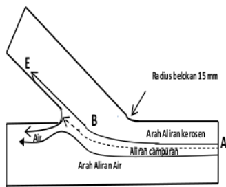
Gambar 6. Skematik aliran untuk kondisi terbaik pada Gambar 5.
