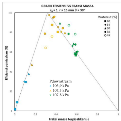
Gambar 9. Hasil Pemisahan fase terbaik pada ( r_D = 1 ), radius belokan 15 mm, sudut 30^\circ , variasi watercut .
