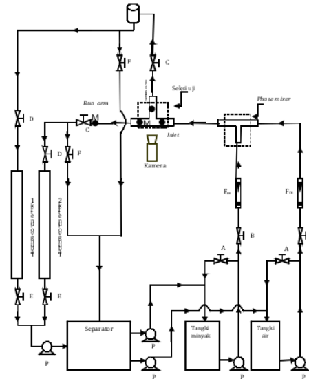
Gambar 4. Skematik peralatan eksperimental
