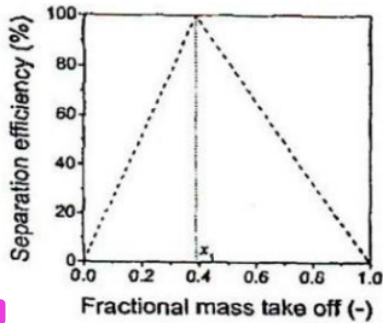
2 Gambar 3. Metode penyajian efisiensi pemisahan dan pemisahan ideal T-junction [9].
