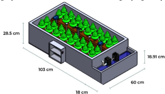
Gambar 3.2 Ukuran Kotak Pertanahan dan Pengairan
