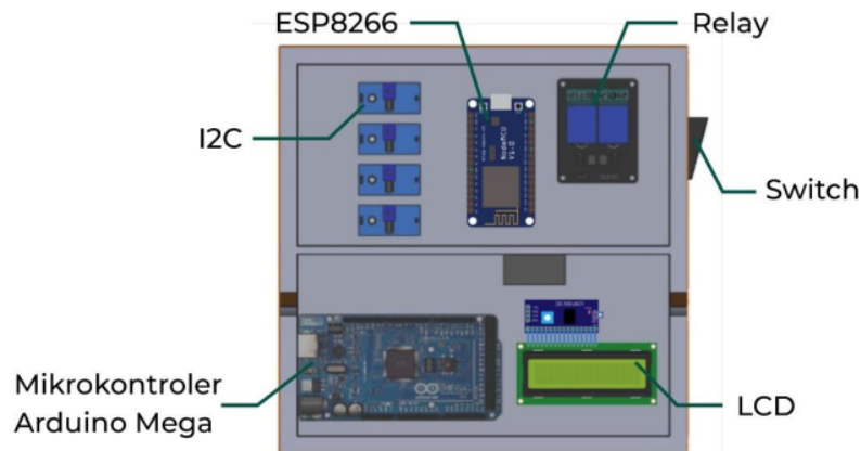
Gambar 2.9 Desain Kotak Panel pada Sistem
