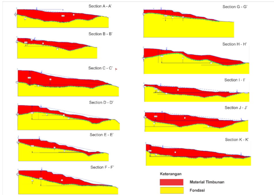
Gambar 5. Geometri disposal berdasarkan section OPD
