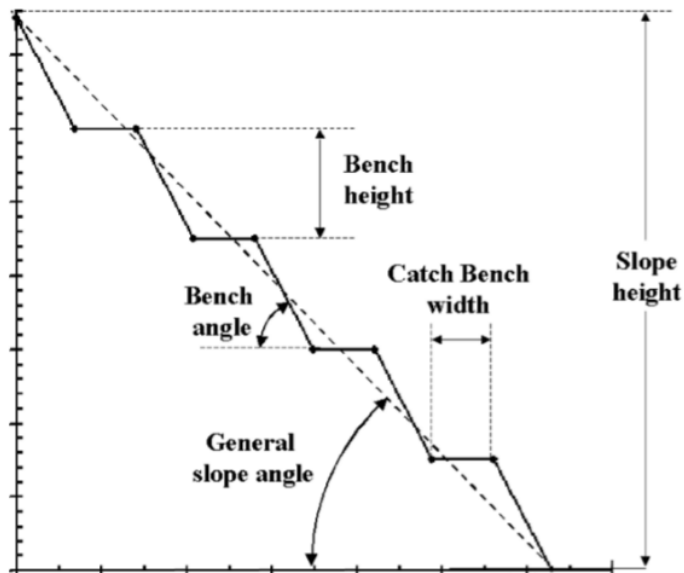
Gambar 3. Geometri lereng tambang (Alejano, 2007)
