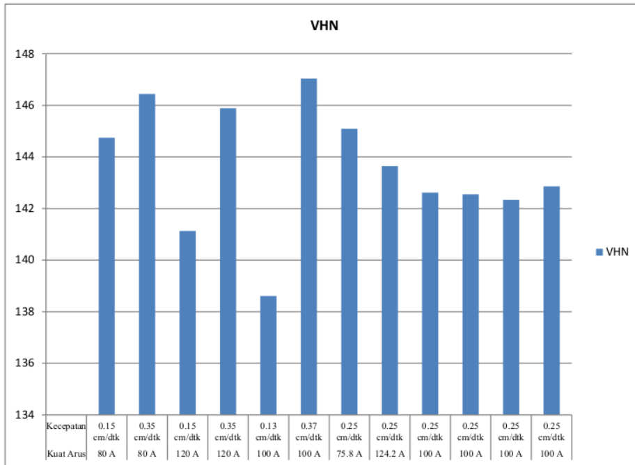
Gambar 7: Grafik Hasil Uji Kekerasan Vickers
