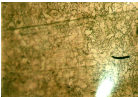
Gambar 17: Daerah HAZ Spesimen dengan arus 124,20 A dan kecepatan 0,25 cm/dtk
