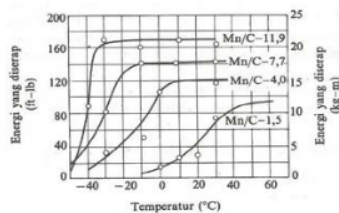
Gambar 1: Pengaruh perbandingan Mn/C terhadap kurva transisi
