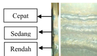
Gambar 4: Pengaruh kecepatan pengelasan terhadap bentuk manik
