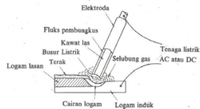
Gambar 3: Las busur dengan elektroda terbungkus
