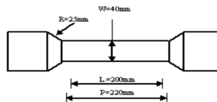
Gambar 6: Spesimen standar JIS
