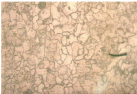
Gambar 21: Daerah HAZ Spesimen dengan arus 100 A dan kecepatan 0,25 cm/dtk
