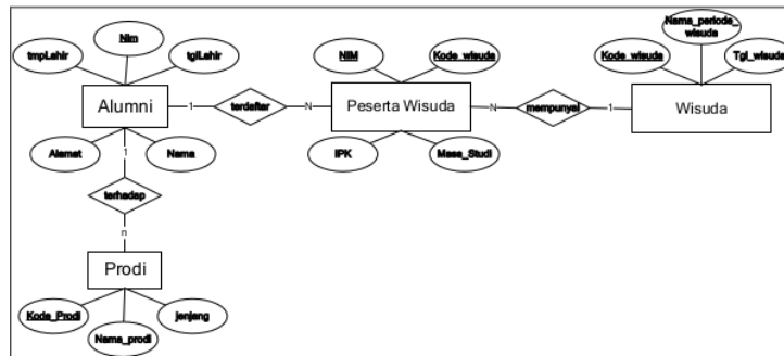
Gambar 2: ERD Pengolahan Data Alumni yang sedang berjalan
