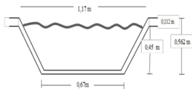
Gambar 2. Bentuk penampang saluran drainase trapesium
