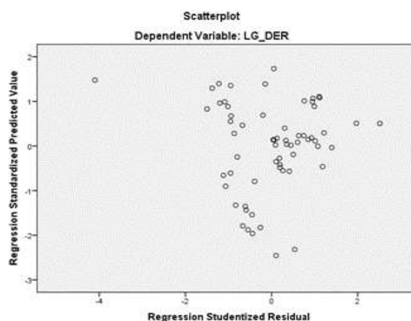
Gambar 1 Uji Heteroskedastisitas
