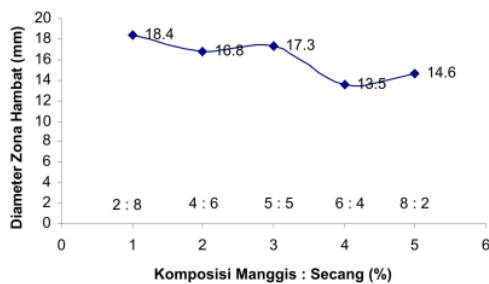
GAMBAR 3: Grafik uji aktivitas antibakteri pada campuran ekstrak terhadap B. cereus
