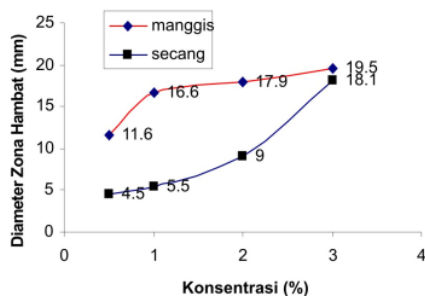
GAMBAR 1: Grafik uji aktivitas ekstrak kering manggis dan secang terhadap B. Cereus
