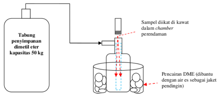
Gambar 1. Ilustrasi perendaman sampel karet dalam DME
