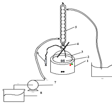
Gambar 3. Rangkaian Reaktor Batch Proses Metanolisis
