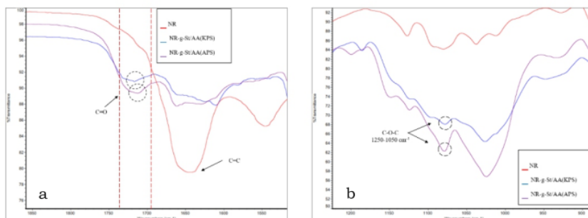
Gambar 4. (a) Spektrum FTIR yang menunjukkan puncak untuk gugus fungsi C=O pada sample NR-g-St/AA dengan inisiator KPS dan sample NR-g-St/AA dengan inisiator APS, (b) spektrum FTIR yang menunjukkan puncak untuk gugus fungsi C-O-C pada sample NR-g-St/AA dengan inisiator KPS dan sample NR-g-St/AA dengan inisiator APS
