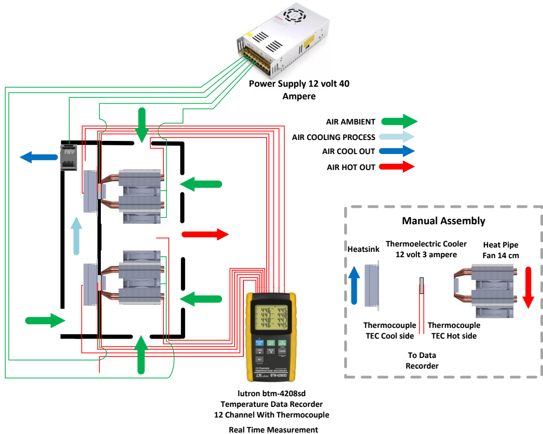
Gambar 7.7 Desain peralatan pengujian dan pemasangan peralatan ukur
