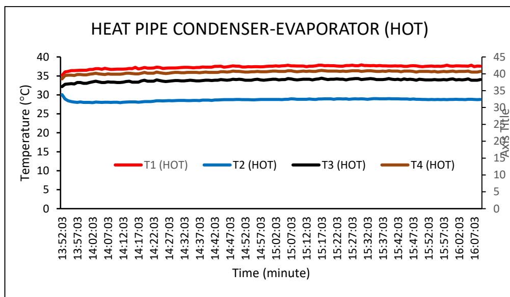
Gambar 7.4 Kurva Temperatur dan waktu ( HOT )
