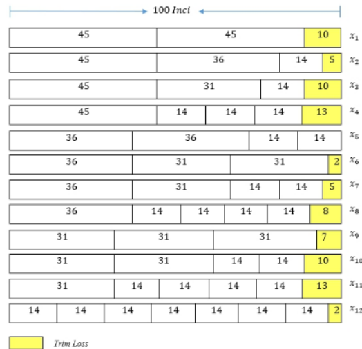
Gambar 1. Kombiasi Pola Pemotongan Layak Lebar Gulungan 100 Inchi dari Sejumlah Permintaan Gulungan
