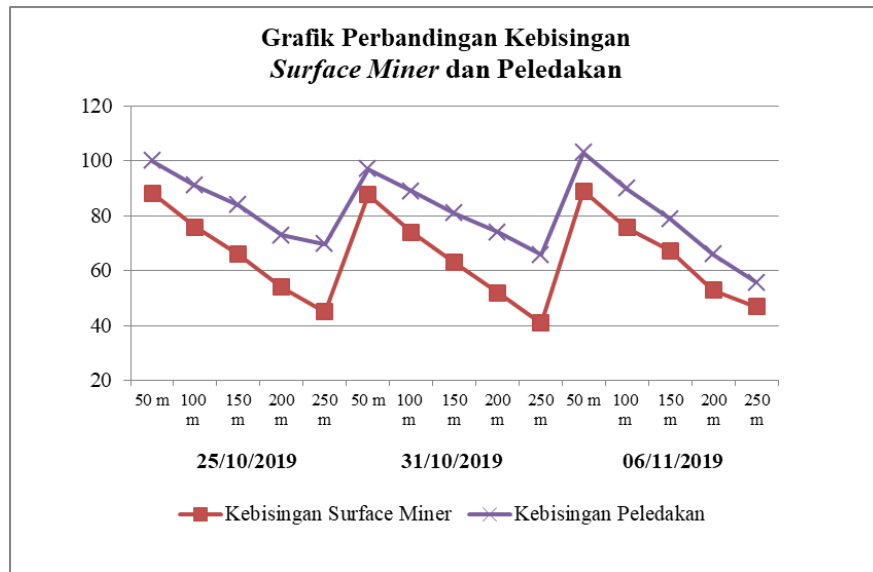
Gambar 6.13 Grafik Perbandingan Kebisingan Surface Miner Dan Peledakan
