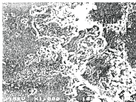
GAMBAR 2: Foto SEM Poliblend setelah biodegradasi
