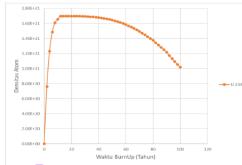
Gambar 6 Perubahan Densitas Atom U 233
