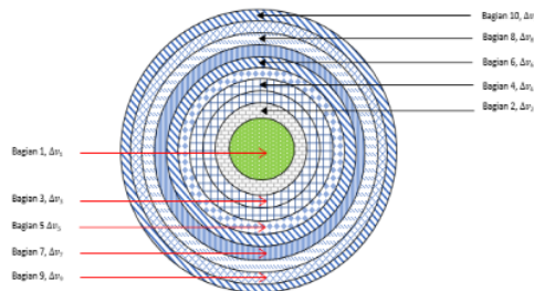
Gambar 3 Skema Modified CANDLE Radial (Tampak Atas)
