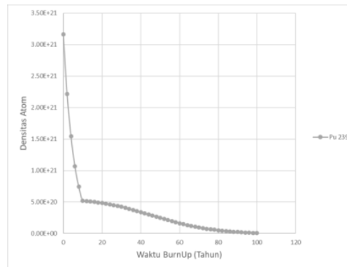
Gambar 7 Perubahan Densitas Atom Pu 239
