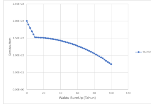
Gambar 5 Perubahan Densitas Atom Th 232
