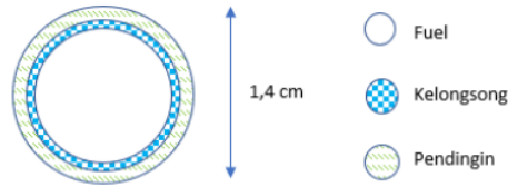
Gambar 1 Geometri Sel Bahan Bakar.
