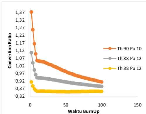
Gambar 8 Nilai Conversion Ratio dalam waktu 100 Tahun
