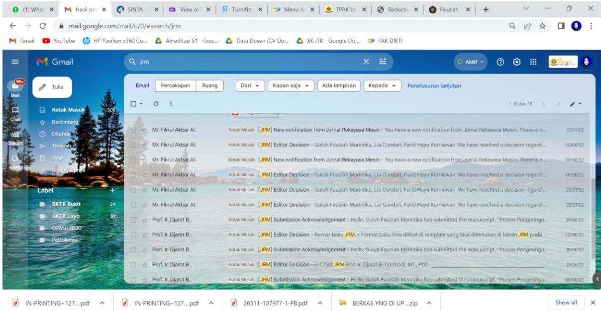
Gambar 1. Daftar Komunikasi-1
