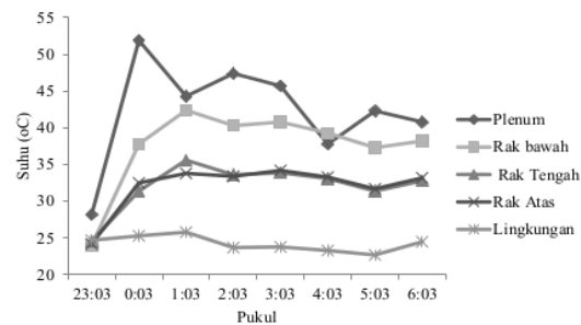
Gambar 3. Distribusi suhu pengering gabah dengan energi biomassa
