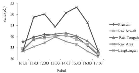
Gambar 2. Distribusi suhu pengering gabah dengan energi surya
