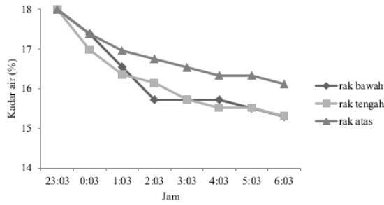
Gambar 6. Grafik penurunan kadar air pengering energi biomassa
