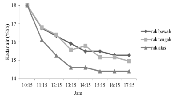
Gambar 5. Grafik penurunan kadar air pengering energi surya
