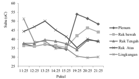
Gambar 4. Distribusi suhu pengering gabah dengan energi kombinasi
