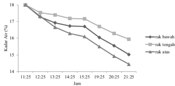
Gambar 7. Grafik penurunan kadar air pengering energi kombinasi
