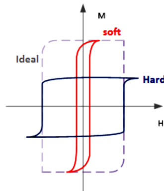
Gambar 3.5. Kurva Histeresis bahan soft dan hard magnets . [21]
