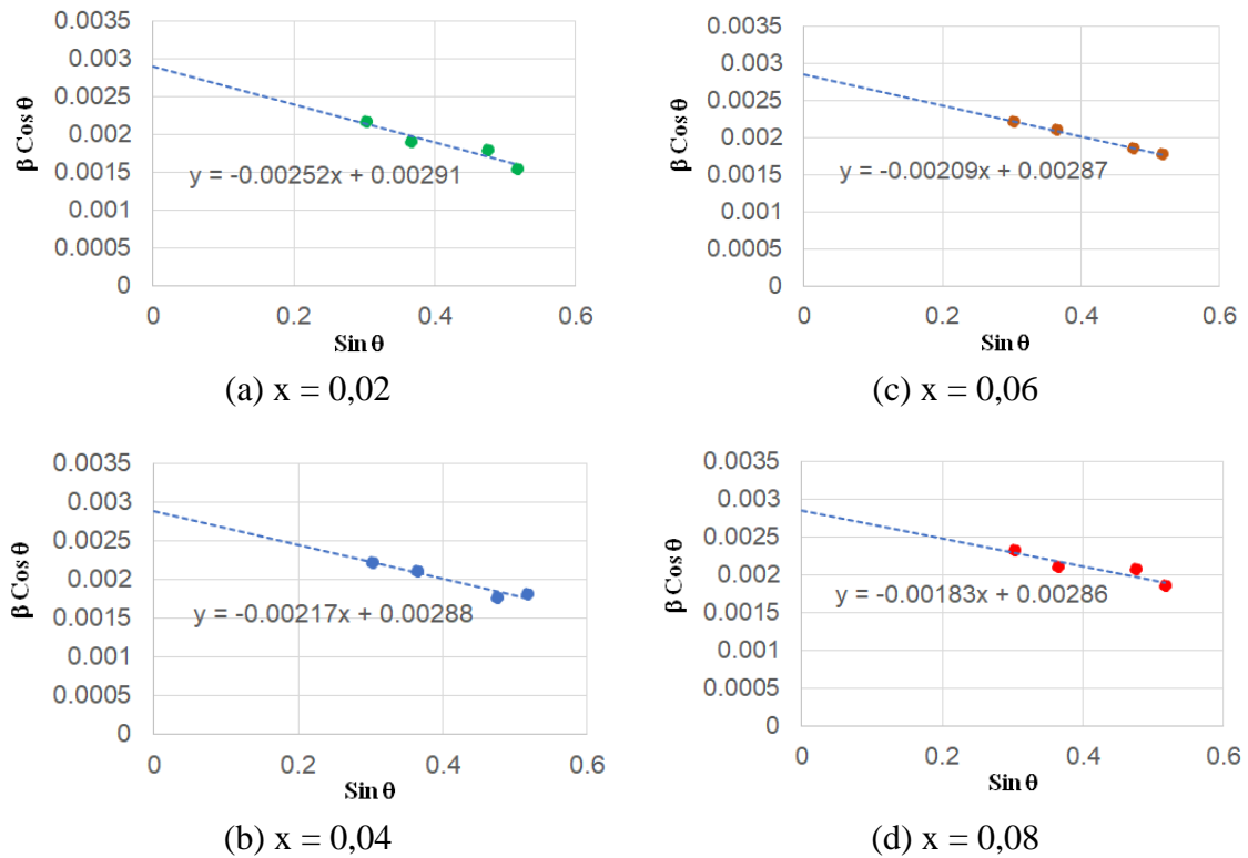
Gambar 5.5. Hasil perhitungan ukuran kristalit menggunakan metode WH
