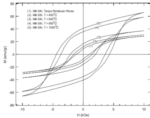
GAMBAR 4: Kurva histeresis bahan serbuk barium heksaferit hasil dari proses milling 30 jam disertai proses annealing pada temperatur 400°C, 600°C, 800°C, dan 1000°C selama 3 jam
