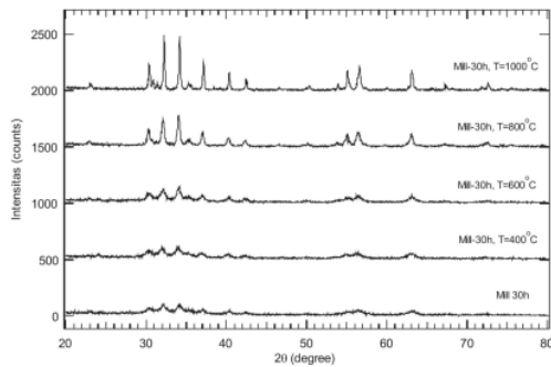
GAMBAR 3: Pola difraksi sinar-X bahan serbuk barium heksaferit dari hasil proses milling 30 jam disertai proses annealing pada temperatur 400°C, 600°C, 800°C, dan 1000°C selama 3 jam
