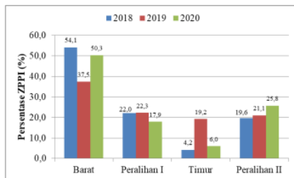
Gambar 6. Grafik rata-rata ZPPI setiap musimnya tahun 2018-2020
