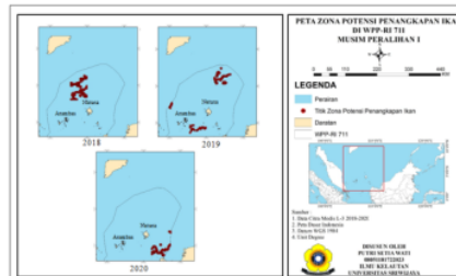
Gambar 3. ZPPI musim peralihan I
