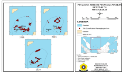
Gambar 2. ZPPI pada musim barat
