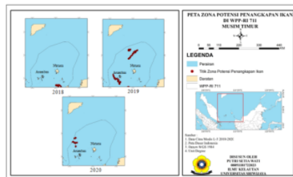
Gambar 4. ZPPI pada musim timur
