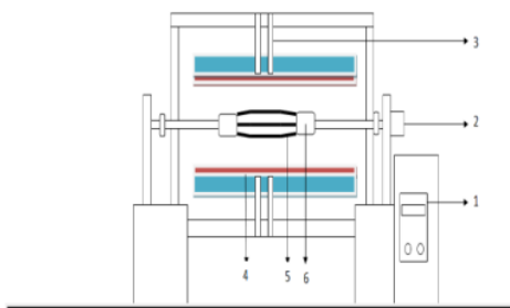
Gambar 1 Rancangan alat pengereng inframerah. 1) Pengatur suhu, kecepatan, dan display kontrol; 2) Motor penggerak; 3) Thermocouple ; 4) Emitter inframerah (1000 watt); 5) Keranjang buah; 6) Stick holder
