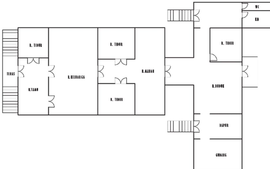
Gambar 3. Denah Rumah Cara Gudang
