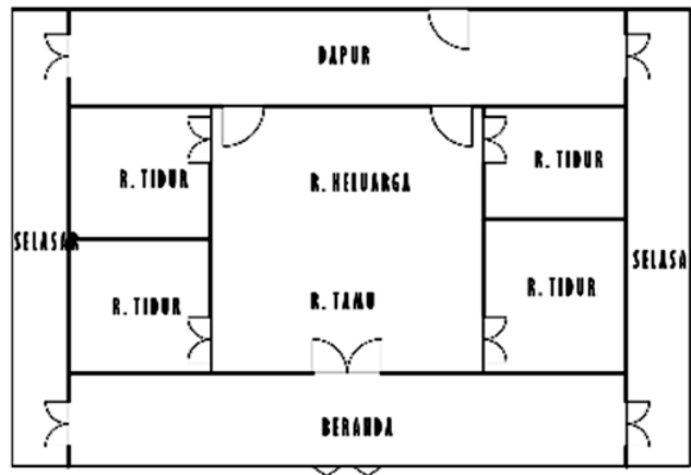
Gambar 4. Denah Rumah Rakit
