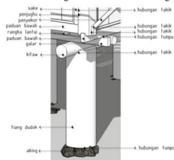
Gambar 4 Hubungan komponen konstruksi bagian bawah Ghumah Baghi
