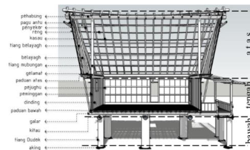
Gambar 2 Komponen konstruksi Ghuma Baghi
