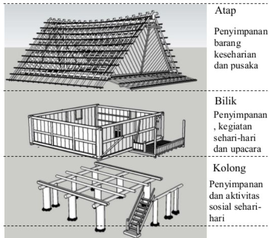
Gambar 1. Pemanfaatan ruang secara vertikal
