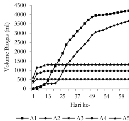
Gambar 3. Akumulasi biogas.
