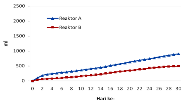
Gambar 9. Grafik akumulasi volume produksi metana
