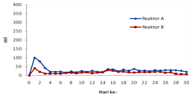
Gambar 10. Grafik pembentukan metana per hari.
