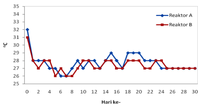
Gambar 2. Grafik suhu pada reaktor.
