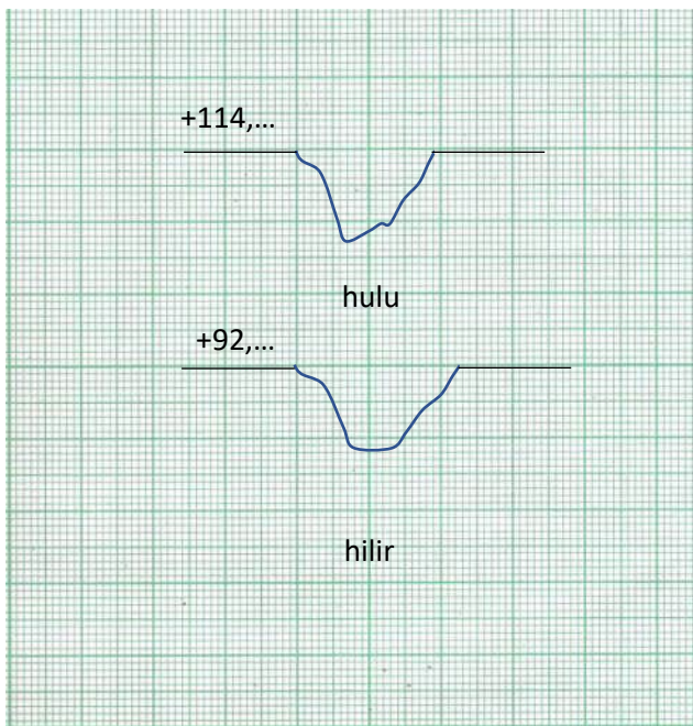
Ruas saluran 17
