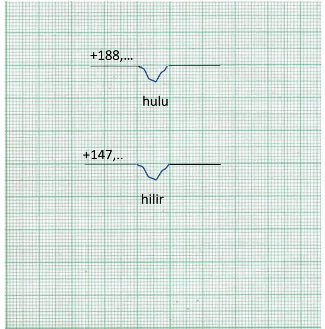
Ruas saluran 4
