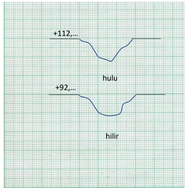
Ruas saluran 18
