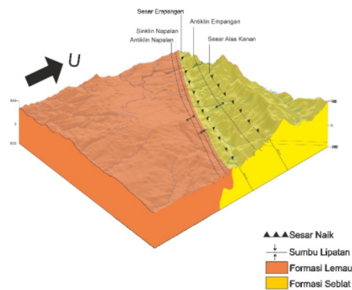
Gambar 5. Model penampang daerah penelitian
