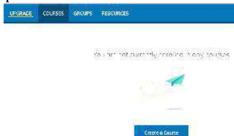
Gambar 45 Pembuatan kelas
