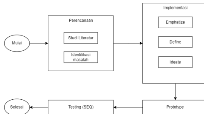
Gambar 1. Tahapan Penelitian
