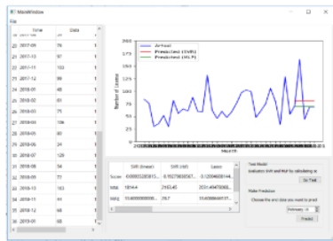
Gambar 7. Hasil SVR dan MLP Dataset 2 menggunakan Bahasa Program Python
