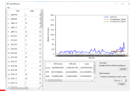
Gambar 6. Hasil SVR dan MLP Dataset 1 menggunakan Bahasa Program Phyton
