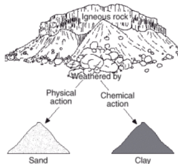
Gambar 4.7. Pelapukan fisik kimia
