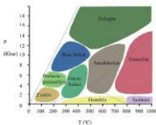
Gambar 4.31. Perubahan struktur metamorfik karena tekanan tinggi
