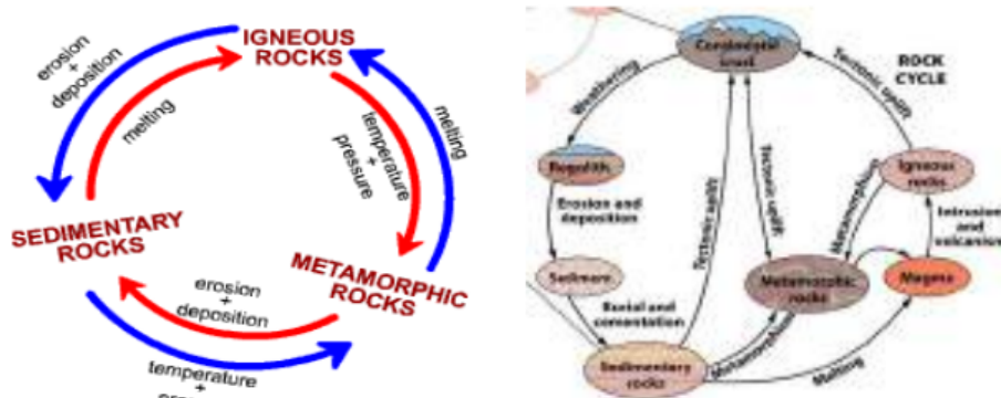
Gambar 4.32. Siklus batuan di alam
