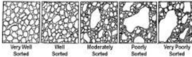
A (Tingkatan sortasi oleh media transpor pada sedimen)
