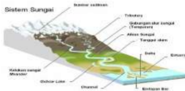
Gambar 4.19. Gambaran umum system sungai
