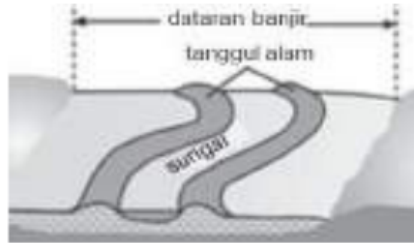
B (Tanggul (www.e-dukasi.net)
