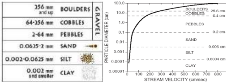
A (Ukuran fraksi material) B (Grafik ukuran fraksi dan aliran)
