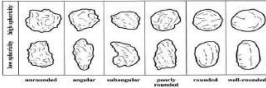
B (Tingkatan pembulatan oleh media transport terhadap batuan)
