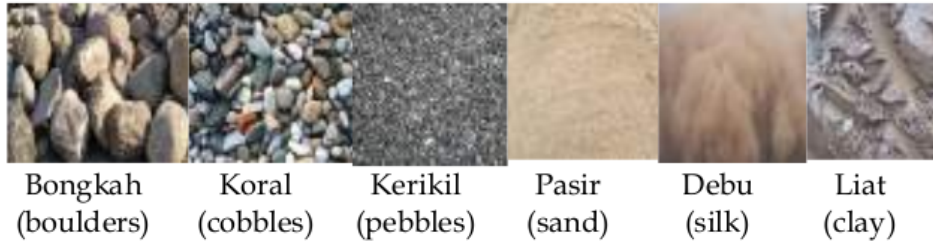
Gambar 4.13. Morfologi ukuran fraksi tanah
