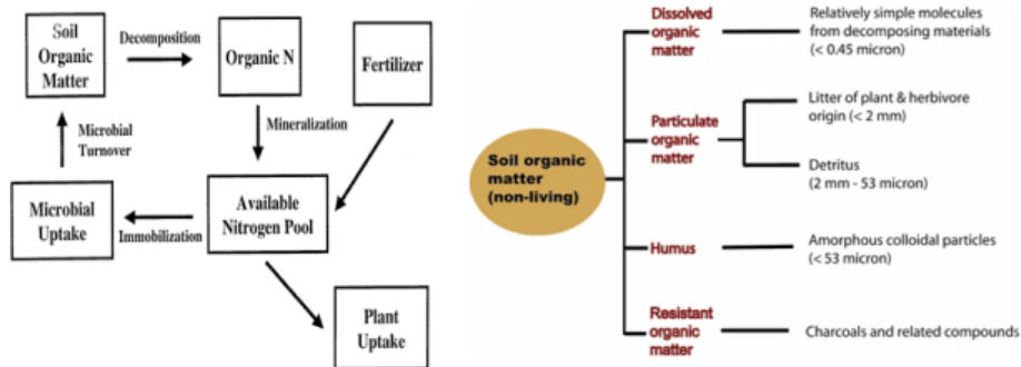
Gambar 9.1 Siklus nitrogen Gambar 9.2. N berasal dari non-living
