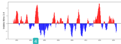
Gambar 3. Grafik Indeks Niño 3.4 tahun 1991 – 2020
