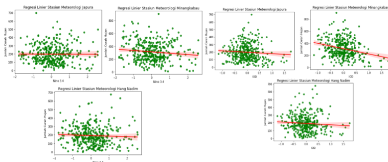
4 Gambar 5. Hasil analisis regresi linier indeks Niño 3.4 terhadap curah hujan
