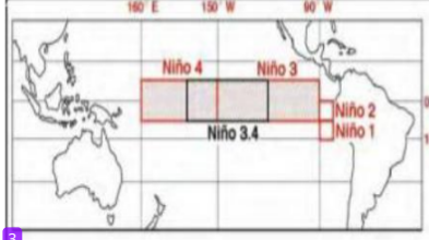
3 Gambar 1. Posisi zona Niño 3.4 di Samudera Pasifik
