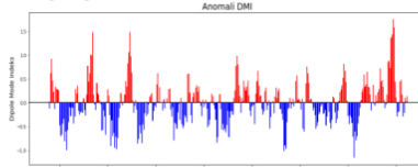
Gambar 4. Grafik Dipole Mode Index tahun 1991 – 2020
