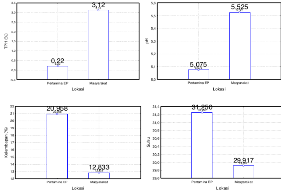
Gambar 2. Rata-rata TPH, pH, kelembaban, dan suhu di lokasi sumur minyak bumi Pertamina EP Asset 1 Field Ramba dan masyarakat
