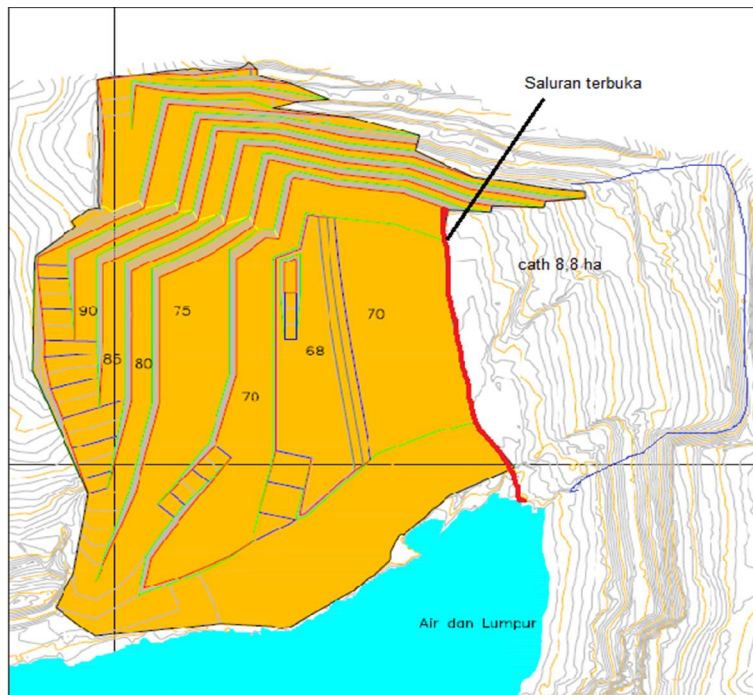
Gambar 4. Posisi Saluran Terbuka
