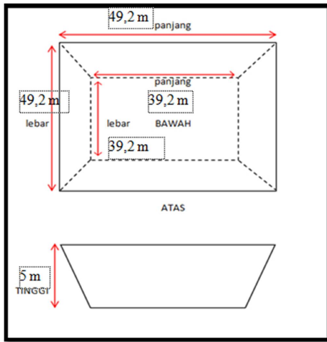
Gambar 2. Dimensi Sump Rencana
