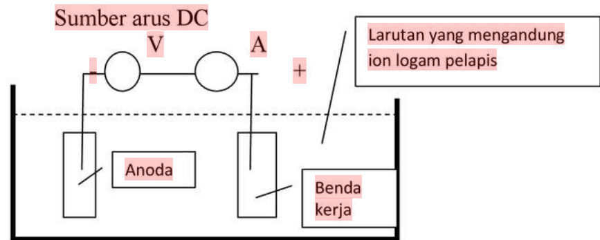
Gambar 11. Diagram kelistrikan proses pelapisan dengan elektroplating
