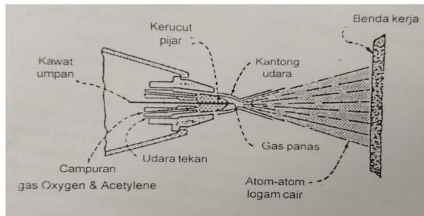
Gambar 6. Anatomi pistol dimana logam pengumpan berbentuk kawat.
