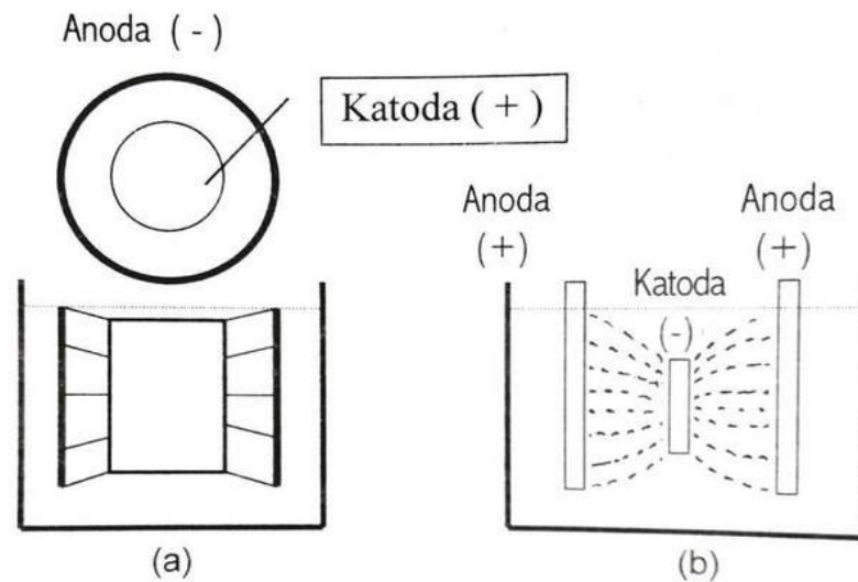
Gambar 13. Distribusi endapan logam pelapis terhadap substrate.
