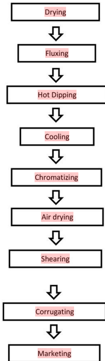
Gambar 1. Diagram alir pelapisan Zn dengan metode celup panas
