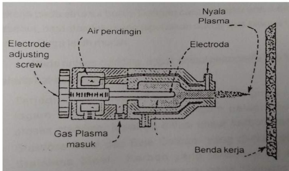
Gambar 9. Anatomi pistol dimana logam pengumpan berbentuk plasma.
