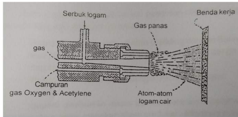
Gambar 7. Anatomi 'pistol' dimana logam pengumpan berbentuk serbuk
