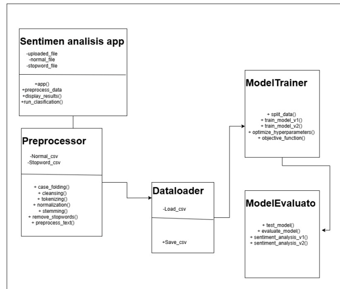
Gambar IV-6.Diagram kelas
