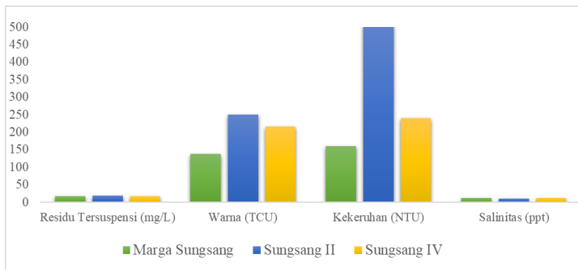
Gambar 3. Grafik kualitas fisik air sungsang sebelum filtrasi
