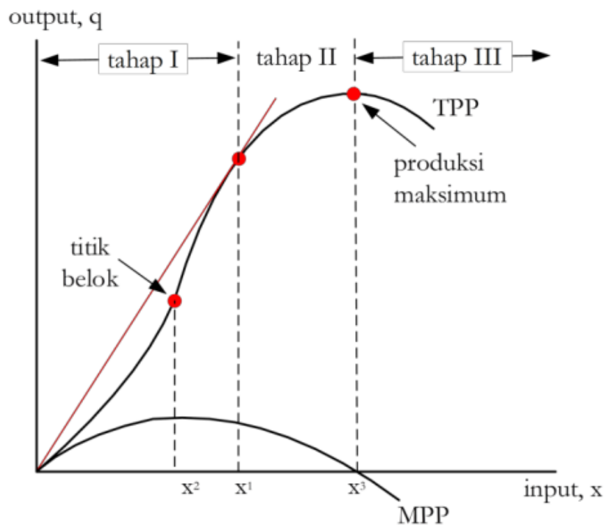
Gambar 7. 1. Kurva produksi neo-klasik
