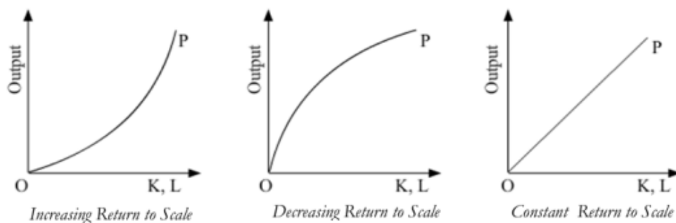
Gambar 6. 1. Tiga tahapan fungsi produksi
