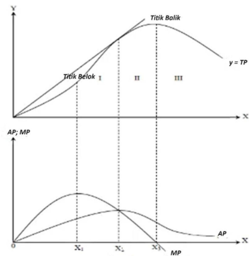
Gambar 6. 2. Hubungan TP, AP, dan MP
