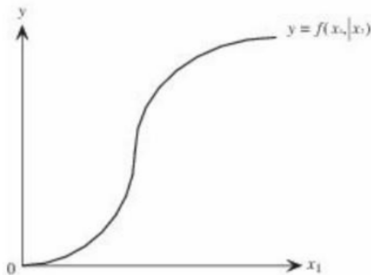
Gambar 11. 1. Kurva Produksi Total
