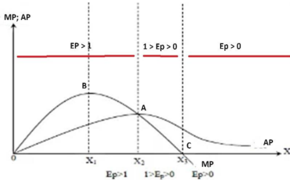
Gambar 6. 3. Hubungan antara elastisitas produksi, MP dan AP
