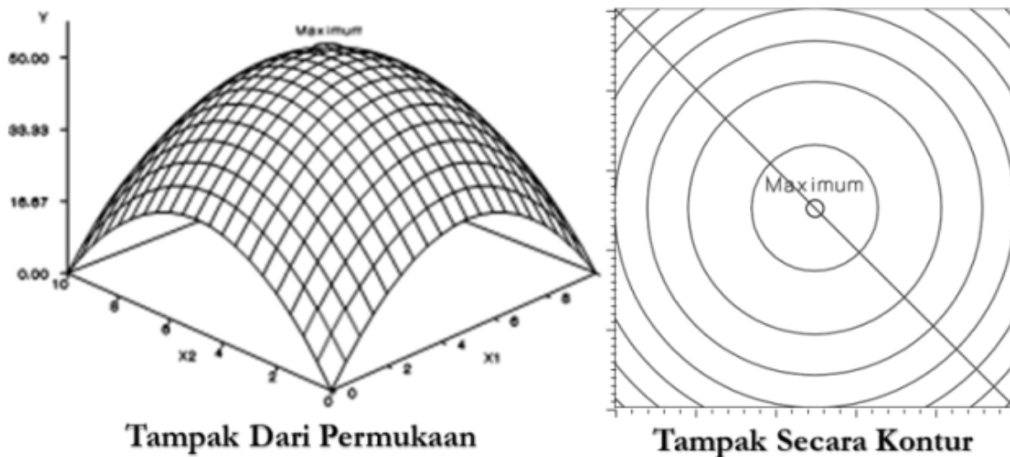
Gambar 9. 1. Ilustrasi Tingkatan Isokuan hingga Titik Maksimum
