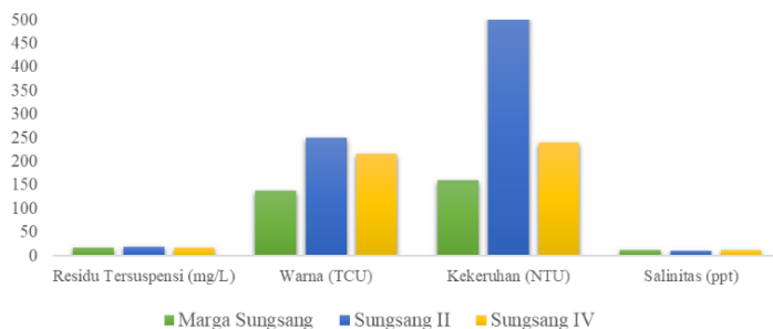
Gambar 3. Grafik kualitas fisik air Sungang sebelum filtrasi
