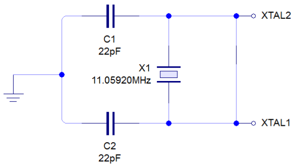
Gambar 3. Rangkaian Oscillator
