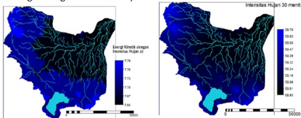
Gambar 2. Intensitas hujan ( I_{30} ) wilayah sub DAS Komerling bagian hulu untuk periode ulang 2 tahun dan Energi Kinetik yang ditimbulkan.
