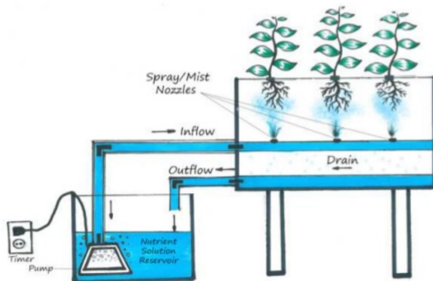
Gambar 36. Sistem Aeroponik
