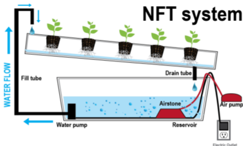
Gambar 31. Sistem NFT
