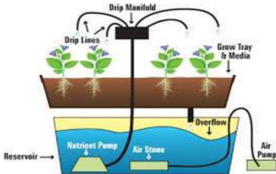
Gambar 33. Sistem Irigasi Tetes Putar (rotasi)
