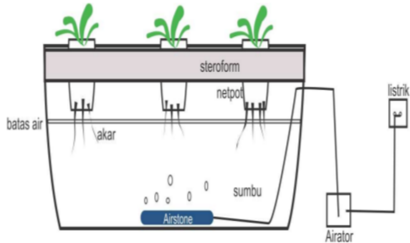
Gambar 30. Sistem Rakit Apung
