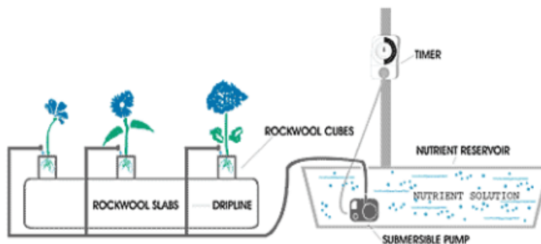
Gambar 34. Sistem Irigasi Tetes Statis (Nonsirkulasi)
