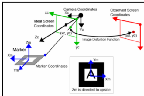
Gambar 9. Sistem Koordinat pada ARToolkit [9]
