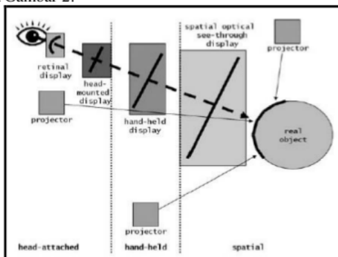
Gambar 2. Pembentukan Objek Virtual pada Sistem Display AR [4]
