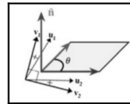
Gambar 10. Vektor v_1, v_2 dan u_1, u_2
