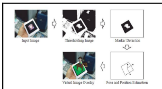
Gambar 5. Aliran Proses Pendeteksian Marker pada ARToolkit [9].
