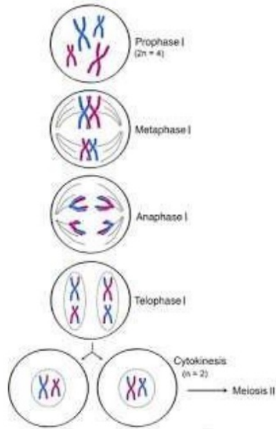
Meiosis I
