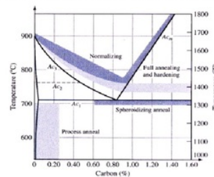
Gambar 2. Kurva Perlakuan Panas
