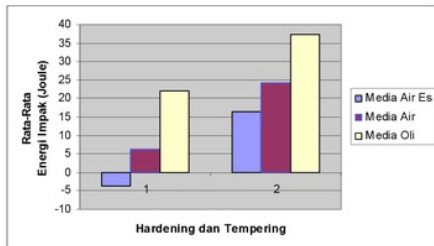
Gambar 7. Hardening dan Tempering pada beberapa media
