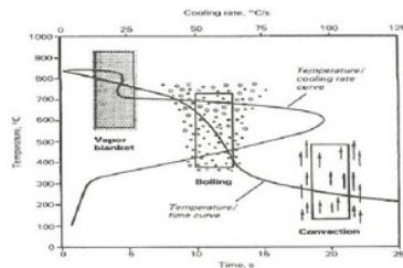
Gambar 3. Mekanisme Pendinginan Dengan Media Cair.
