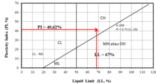
Gambar 3. Grafik plastisitas untuk klasifikasi tanah
