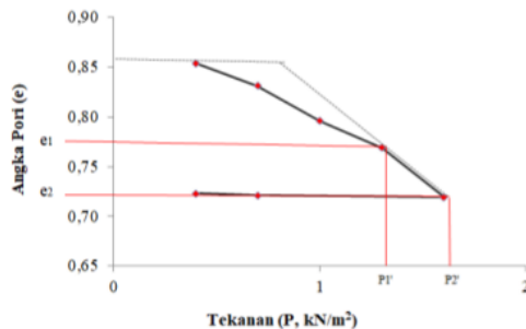
Gambar 7. Kurva hubungan e-log P
