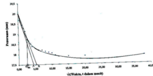
Gambar 6. Metode Akar Waktu/Taylor
