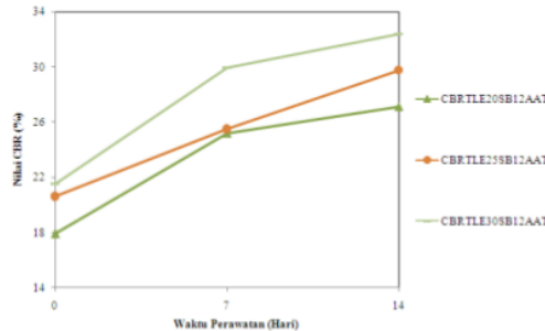
Gambar 11. Grafik nilai CBR 12 % AAT dan variasi SB
