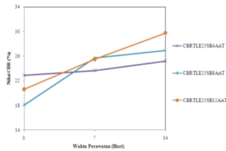
Gambar 7. Grafik nilai CBR 25 gr/liter air SB dan variasi AAT
