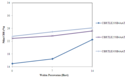
Gambar 9. Grafik nilai CBR 4 % AAT dan variasi SB
