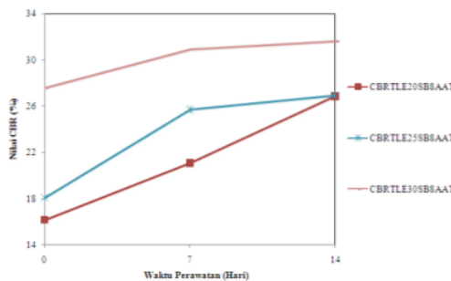
Gambar 10. Grafik nilai CBR 8 % AAT dan variasi SB
